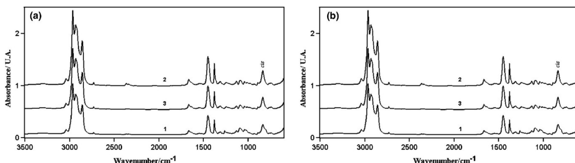
Hình 2. Phổ FT-IR của cao su thu được từ giống thương mại PB 235 (a) và từ cây rừng tại lối đi rừng Carauari (b), sử dụng ba loại chất đông tụ: (1) axit formic, (2) axit khối và (3) axit axetic.
